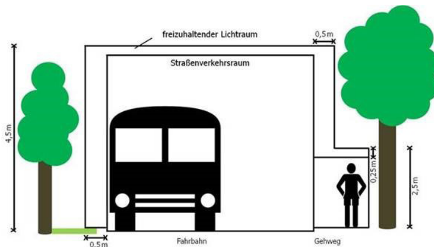
Grafik: Straßenlichtraumprofil, das von Bewuchs freizuhalten ist
